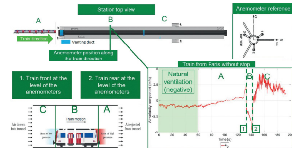
Illustration schématique de l'effet piston mesuré à Sevran-Beaudoctes montrant l'évolution de la vitesse d'air pendant le passage d'un train.
