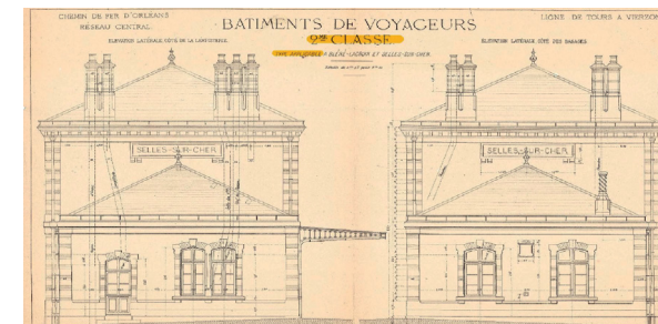
Plan-type des BV de 2 e classe de La Compagnie du chemin de fer de Paris à Orléans.
