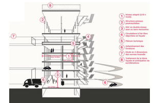
Principes architecturaux et techniques d'un bâtiment mixte. © AREP, 2024
