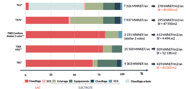
Répartition des usages énergétiques annuels par technicentre (chauffage, ECS, éclairage, équipements). © AREP, 2024
