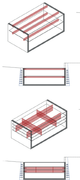
Solutions et variantes de butonnement explorées. © AREP, 2024
