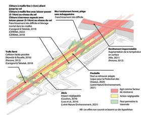
Détail des formes architecturales et leurs effets sur le mouvement potentiel de la faune à l'échelle de la gare.
